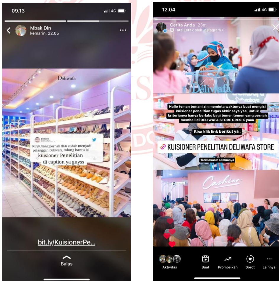
Gambar 2 Penyebaran Kuisioner
